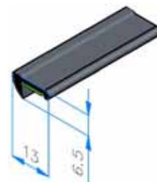
Coprigiunta Joint cover
